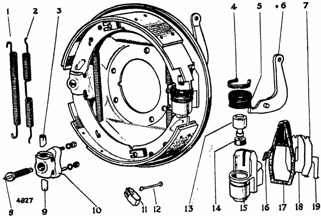
Fig. 5. Vue éclatée d'un frein arrière.
