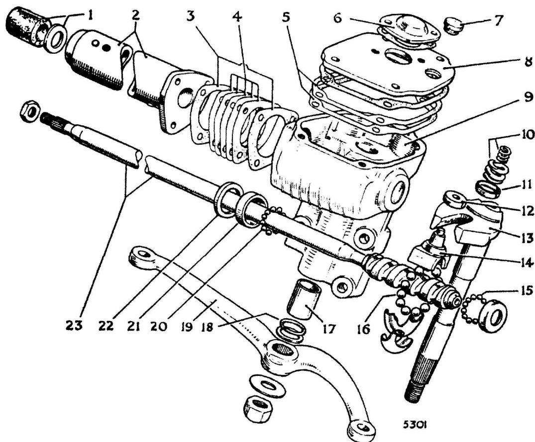
Fig. 1. Vue éclatée de la direction, type 'F'.
